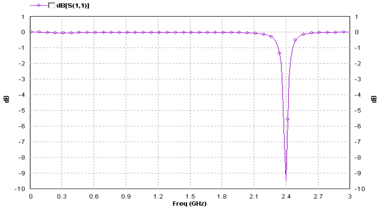
Figure 3. S parameter for 2x1 Antenna Array
